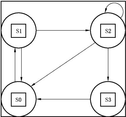
图 B.1 泄漏补偿换气控制系统的状态图示例
