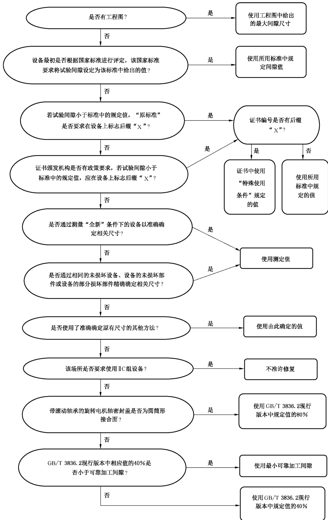
图 D.1 修复部件最大间隙的确定
