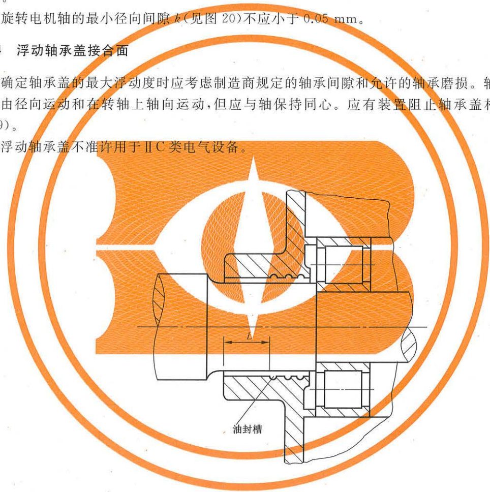
图 17 用于旋转电机轴的圆筒形结合面示例
